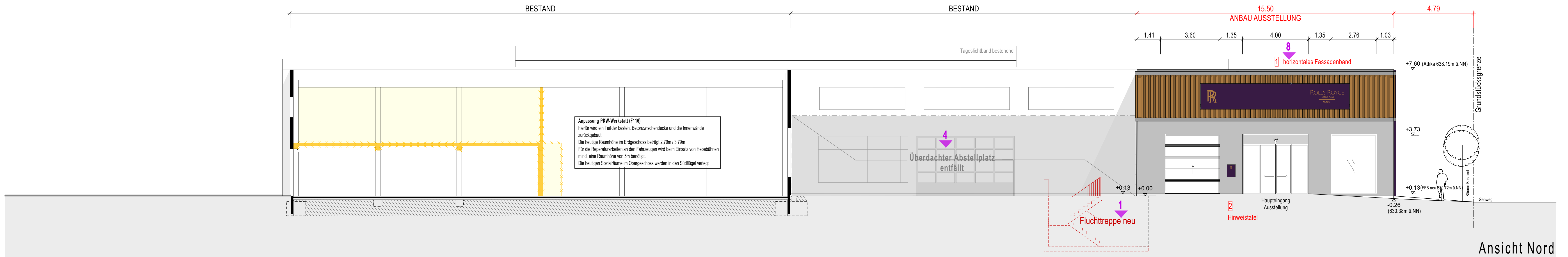
Ansicht Nord Haupteingang Ausstellung
