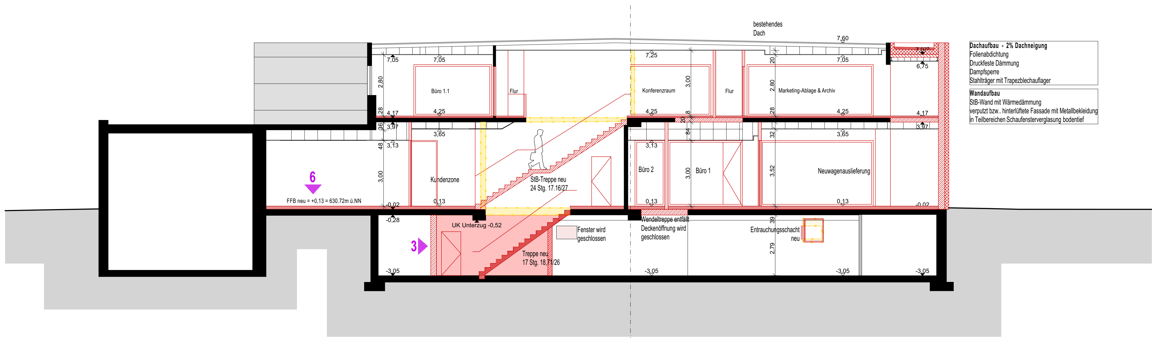
Schnitt 3-3
