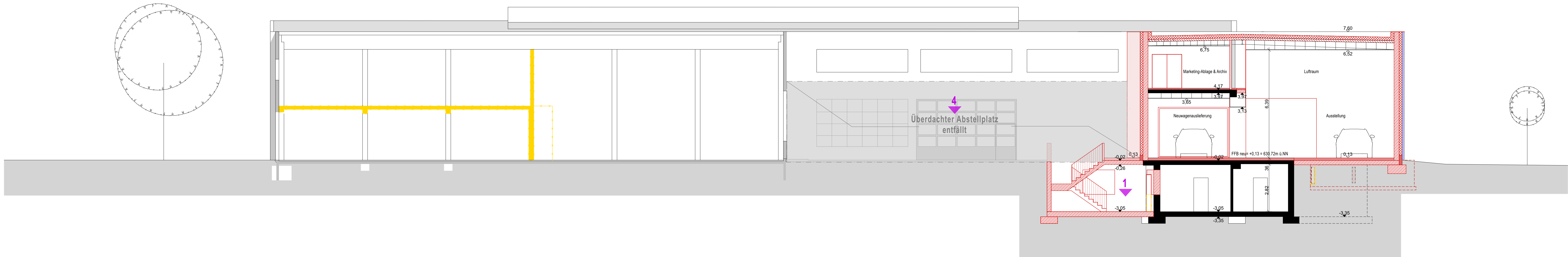
Schnitt 4-4
